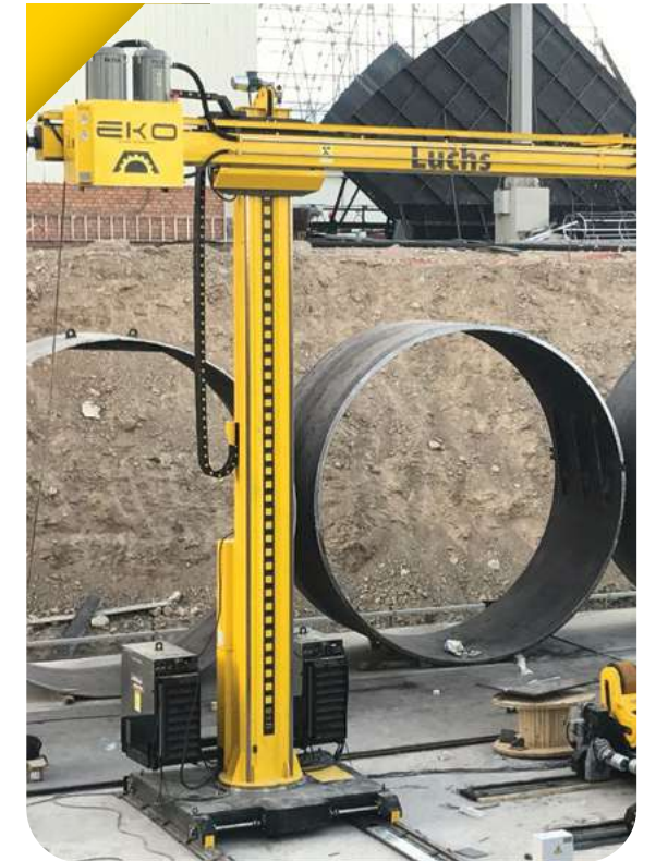
Pozisyonerin hareketiyle dairesel flanş kaynağı
