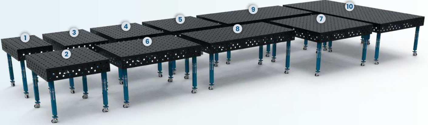
EXPERT, PRO, PLUS ve ECO MASALARIN ÖLÇÜLERİ [mm].
